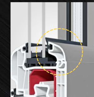
STANDARDGLASLEISTE
